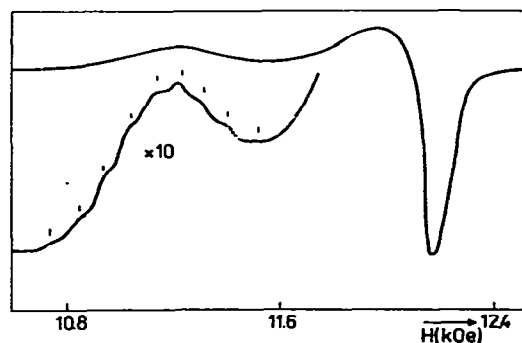
Fig. 9. Q-band ESR spectrum of [\text{Cu}_2(\text{dien})_2(\text{NCO})_2](\text{Bph}_4)_2 \cdot 2 \text{H}_2\text{O} .
